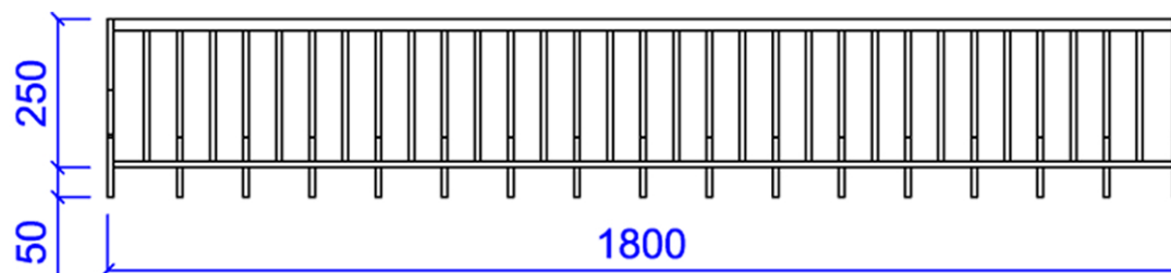
上面図
