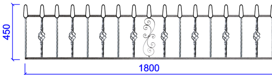
正面図
